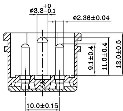
A-A SECTION
